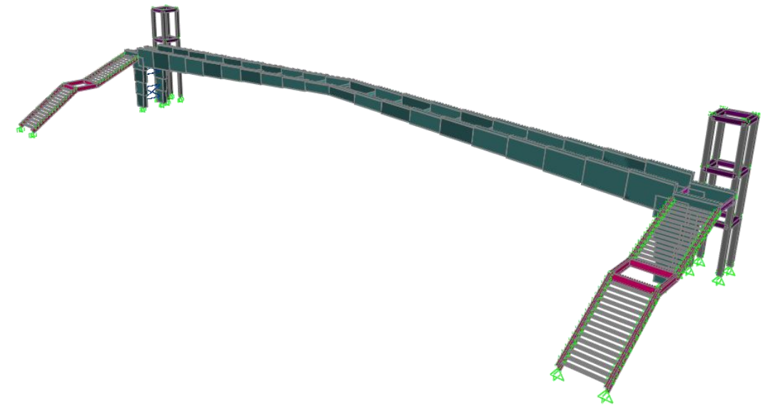
2.- Puente Peatonal CBTIS.
